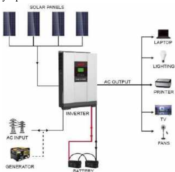
Рисунок 1 Гибридный солнечный инвертор
