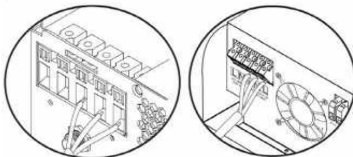
Рисунок 3 Подключение вывода переменного тока
