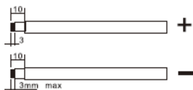
Рисунок 5 Разделка солнечного кабеля
