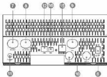
5.2KW модель только с одиночной работой
