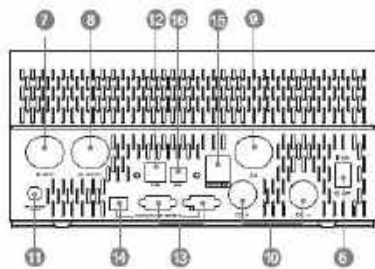
5.2KW модель с параллельной работой
