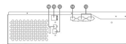
2кВт-5,5кВт исполнение для параллельной работы
